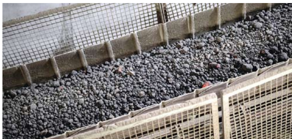
3. attēls. Klinkers tikko pēc transportēšanas no rotācijas krāsns.
